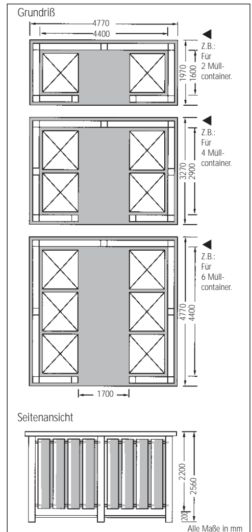
Abb.: 1 Grundeinheit für 4 Großmülltonnen à 1100 Liter, Länge 4,77 m, Tiefe 3,27 m; 2 Seitenwände, 1 Rückwand, 1 Vorderwand rechts, links, 1 Doppelflügeltür verzinkt. Alle Stahlteile feuerverzinkt und pulverbeschichtet (außer Tür) in RAL 6005 moosgrün, Wände mit Holzpaneelen beplankt, Holz imprägniert.
